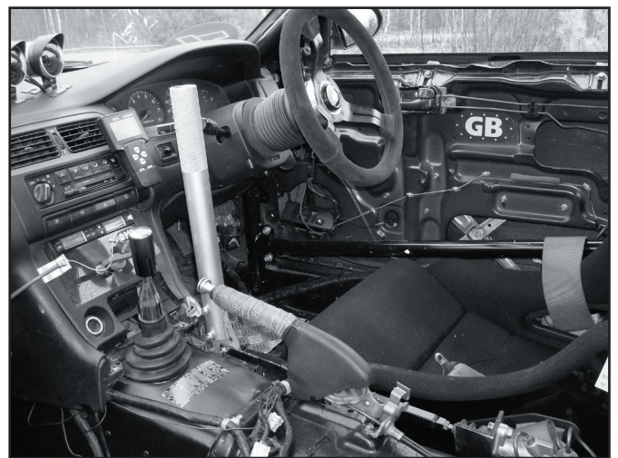
Bilens förarplats.
